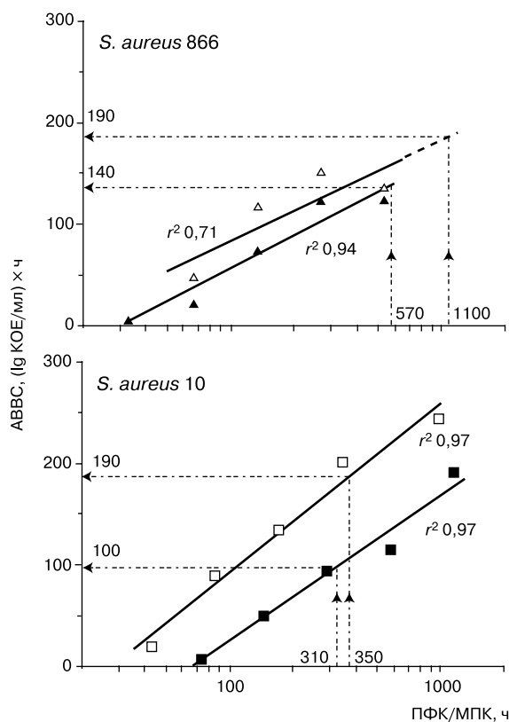
Рис. 3. Зависимость АМЭ даптомицина и ванкомицина в отношении S. aureus от ПФК/МПК. △, □ – даптомицин, ▲, ■ – ванкомицин.
